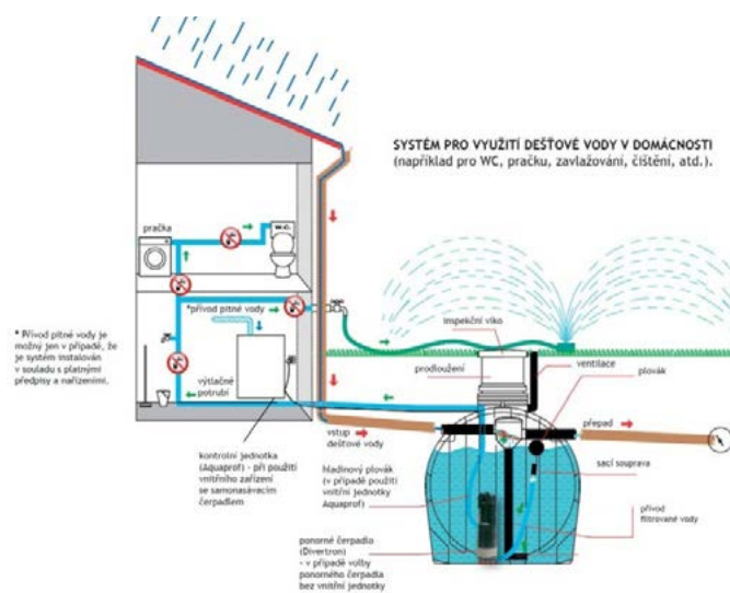
Schéma systému pro využití dešťové vody v domácnosti Zdroj: tzb-info.cz
